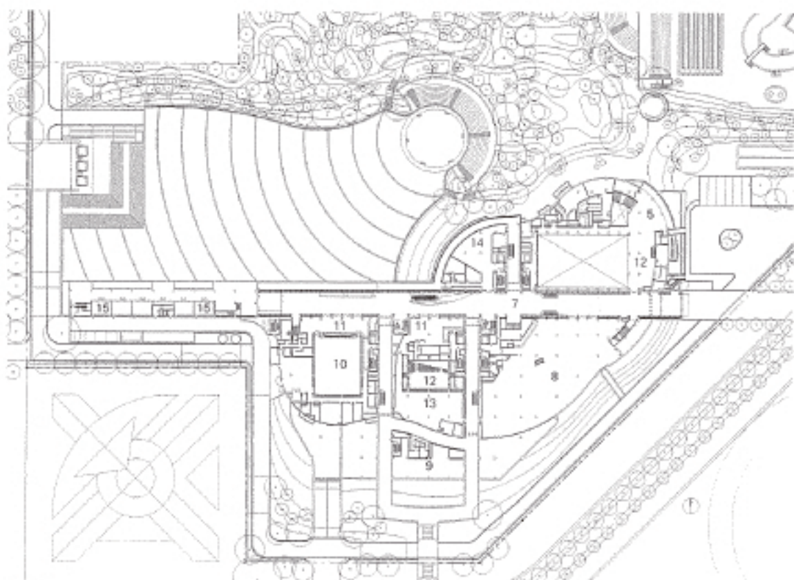
1階平面
